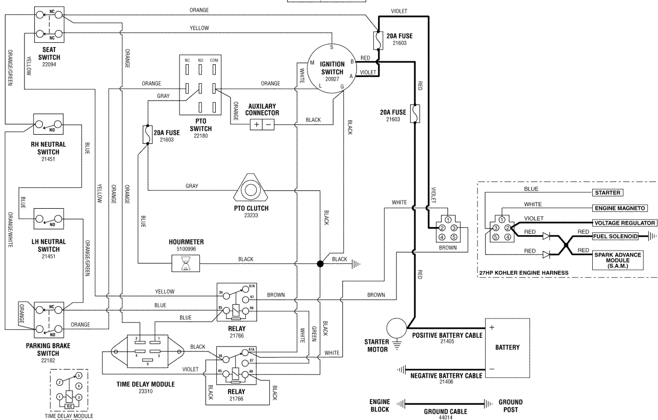
IS3000ZX KOHLER WIRE HARNESS 61826
